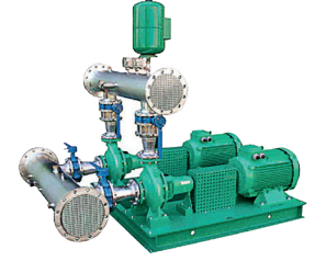
YANGIN HİDROFORU
